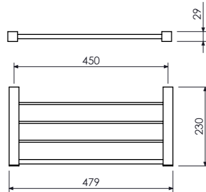
Toalheiro Rack sem Alça Towel Rack without Towel Bar, Rack para Toallas sin Barra Cod. 21.35.084.120.08
