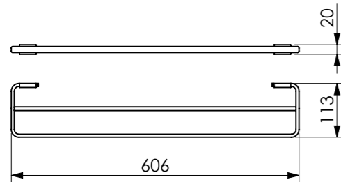
Toalheiro Duplo Towel Ring, Porta Toalla de Argolla Cod. 21.35.069.143.08
