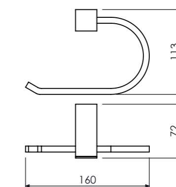
Toalheiro Argola Towel Ring, Porta Toalla de Argolla Cod. 21.35.026.120.08
