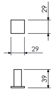
Porta Roupão Robe Hook, Porta-Robe Cod. 21.17.131.120.08
